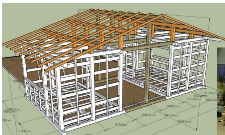
※木造軸組 2/3 模型
